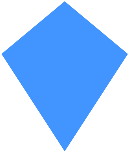
Drachenviereck
