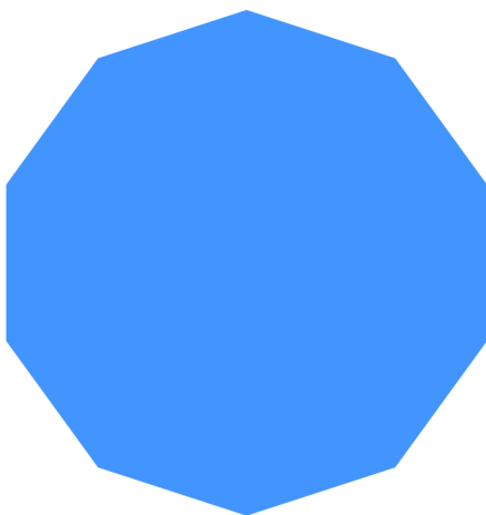
Zehneck (Dekagon)
