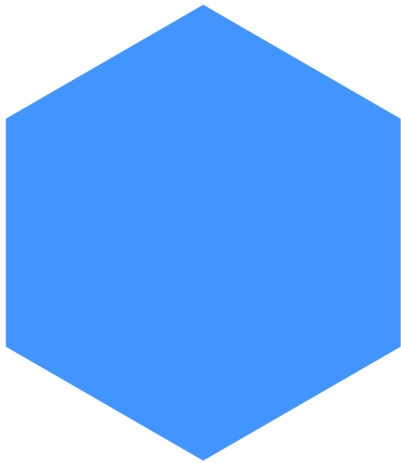
Sechseck (Hexagon)
