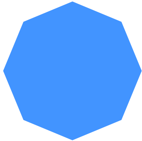
Achteck (Octagon)
