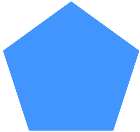
Fünfeck (Pentagon)
