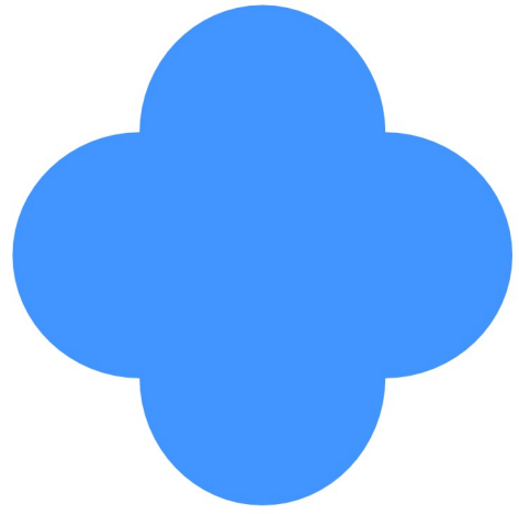
Vierpass
